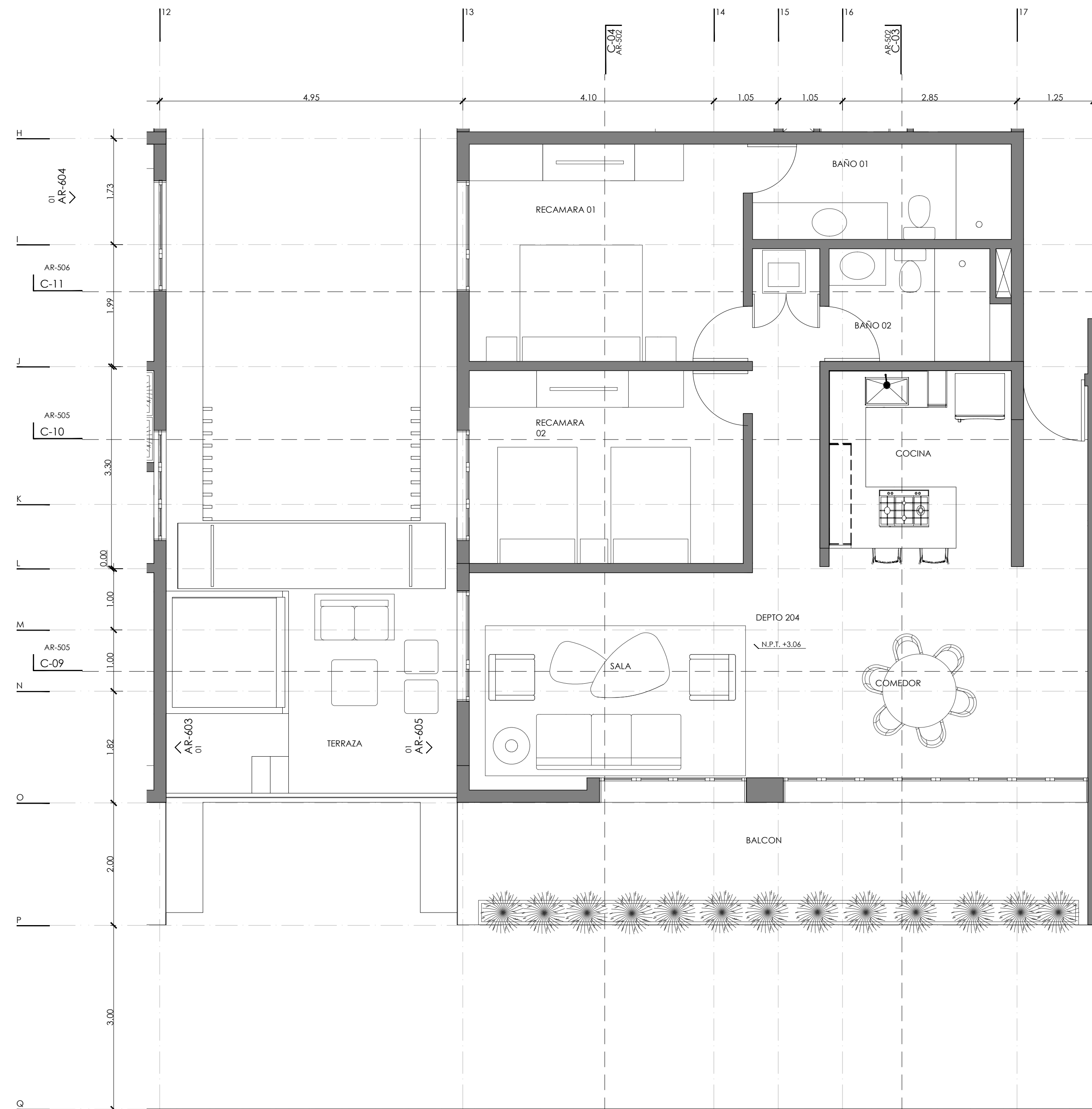
01 PLANTA DEPARTAMENTO 204
